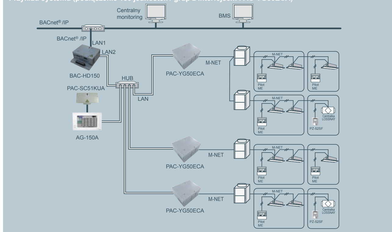
Przykład systemu (podłączenie 150 jednostek / grup z interfejsem PAC-YG50ECA)
